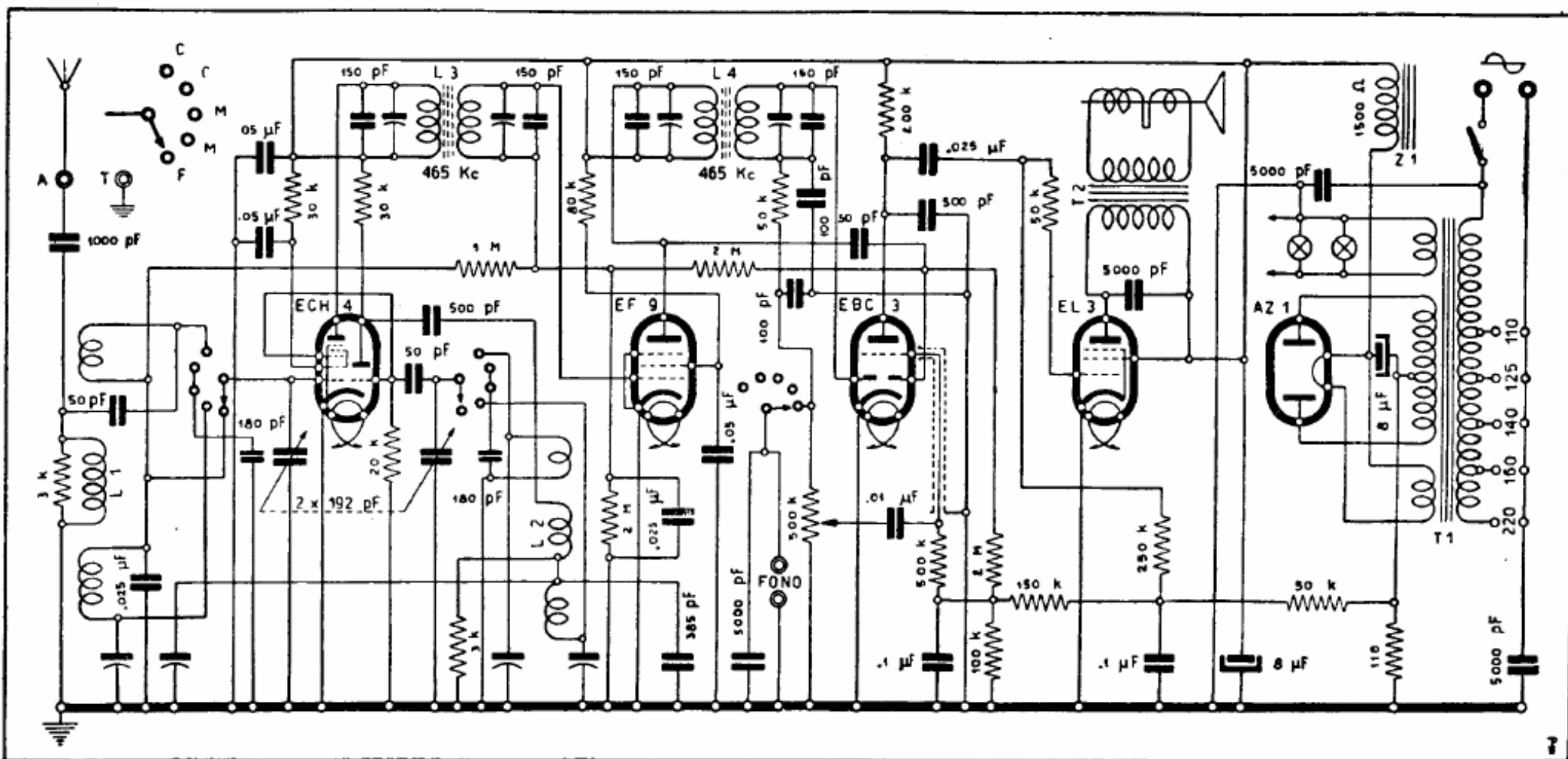
EFFEDIBI' RADIO (F.LLI DE BERNARDI) - Mod. SOAVE - Gamma medie divisa: 187-436 m e 432-570 m. Gamma corte: 17-36 m e 35,5-49 m. Media frequenza: 465 kc. Tensione anodica massima 220 V, schermi 160 V, placca oscillatrice 90 V, griglia finale — 5,6 V, eccitazione 100 V. Resa uscita 3 W, consumo 48 W.
